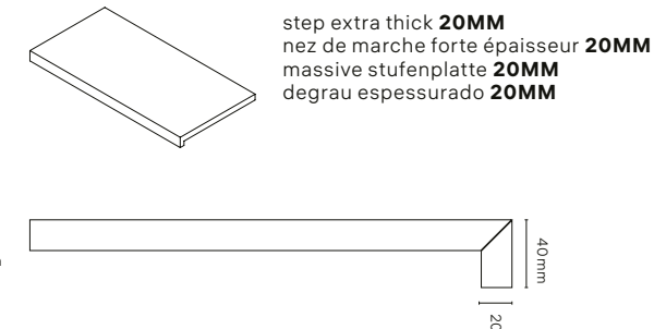
overflow grille 20MM grille 20MM überlauf 20MM grelha 20MM
